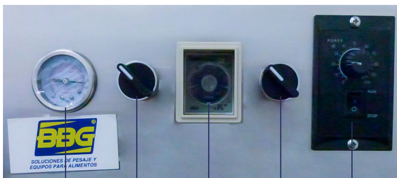
Vacuómetro On / Off Vacío Temporizador On / Off Rotación Regulador velocidad
